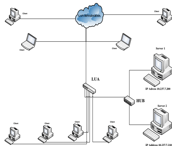
Gambar 4. Rancangan Sistem
